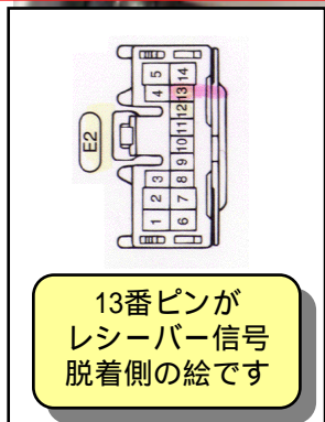
リモコンレーザー信号コネクタ
